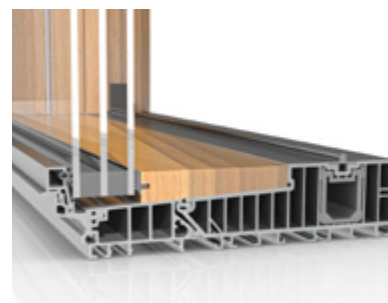
Seitenschnitt mit Verglasung der Hebe-Schiebe-Tür „HST“
