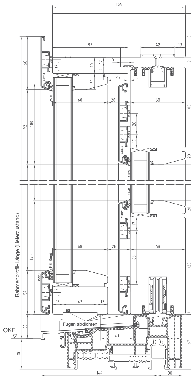
Vertikalschnitt
