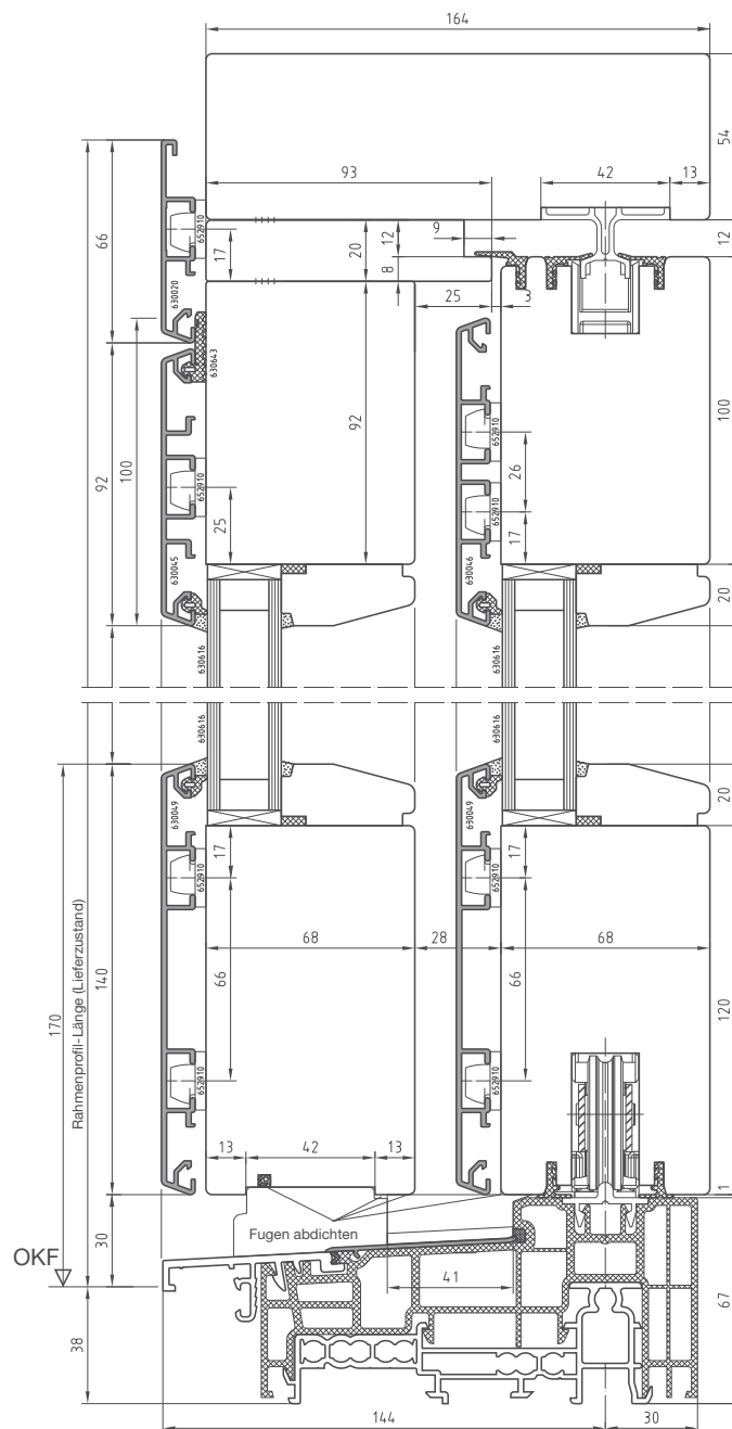
Vertikalschnitt
