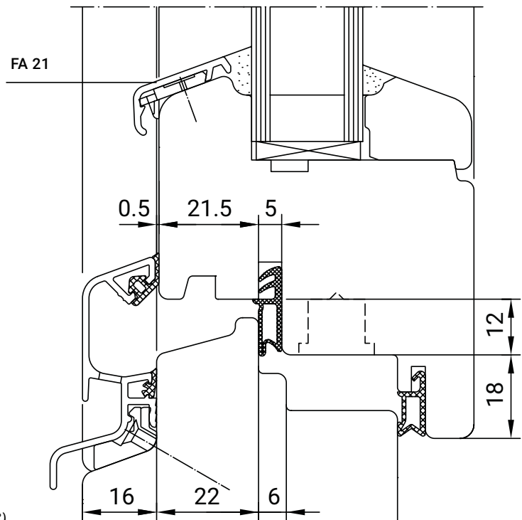
Einbaubeispiel AP 16.23
