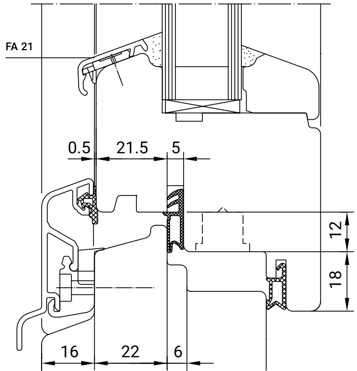
Einbaubeispiel AP 16.24
