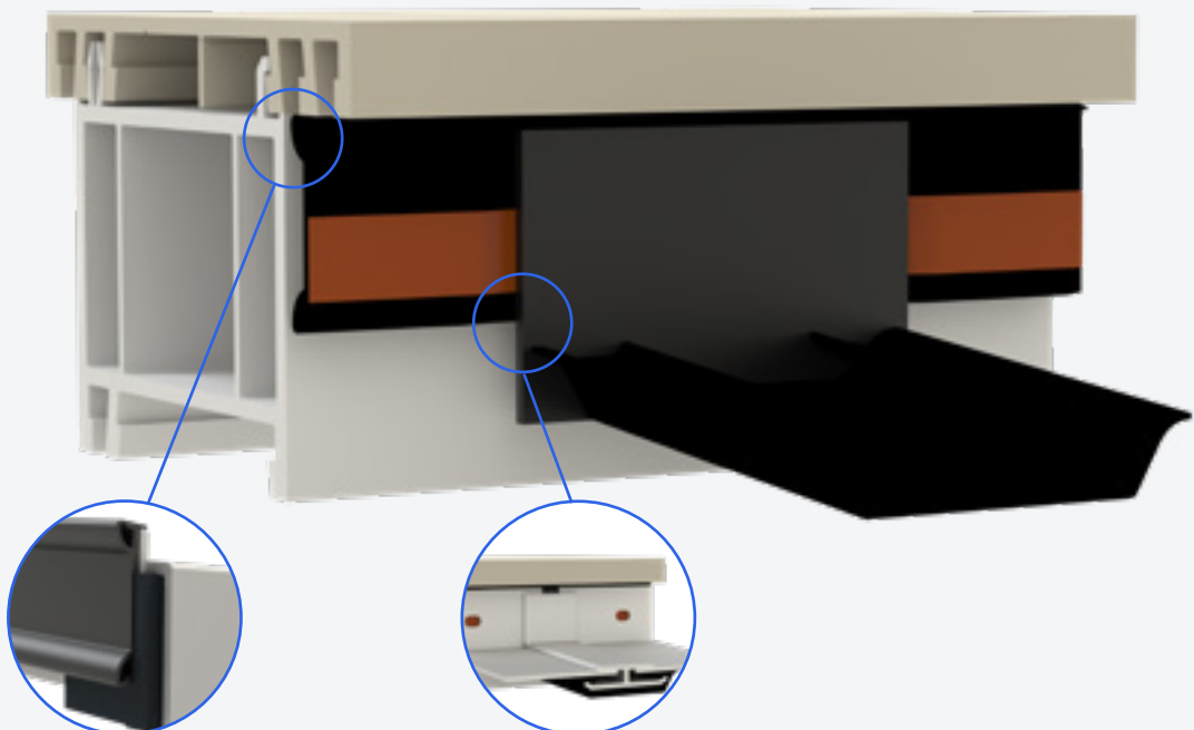
Selbstklebende Anschraubdichtung
