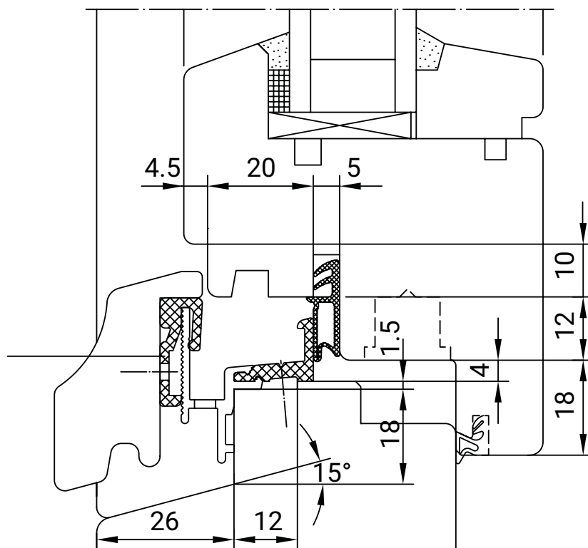
Einbaubeispiel TR 12.25 Stil
