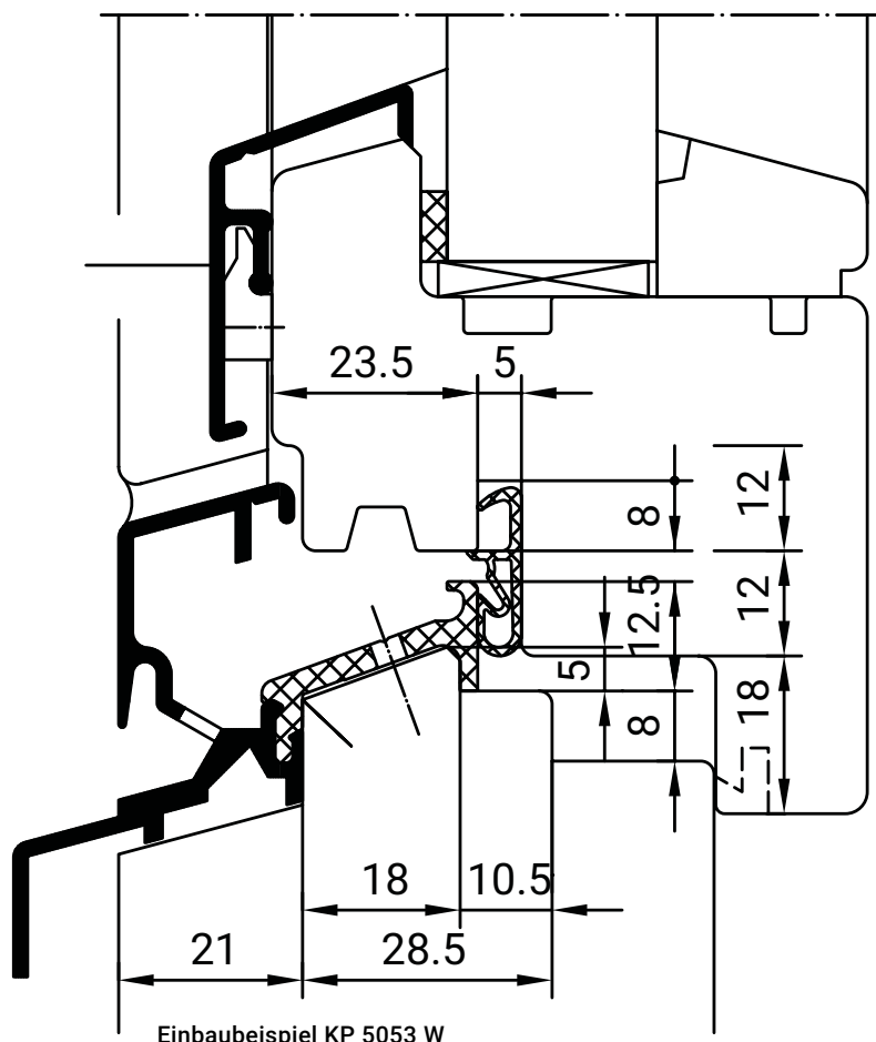
Einbaubeispiel KP 5053 W
