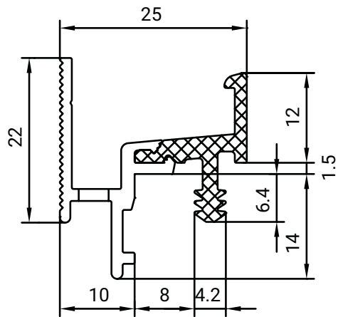
TR 12.25 K Stil
