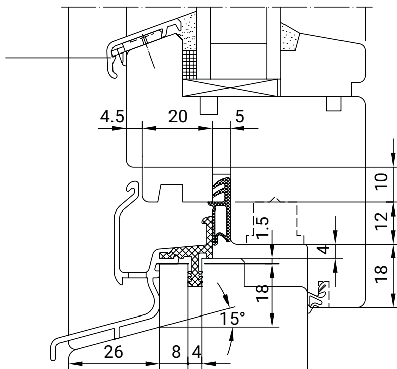
Einbaubeispiel GTR 25.46 K
