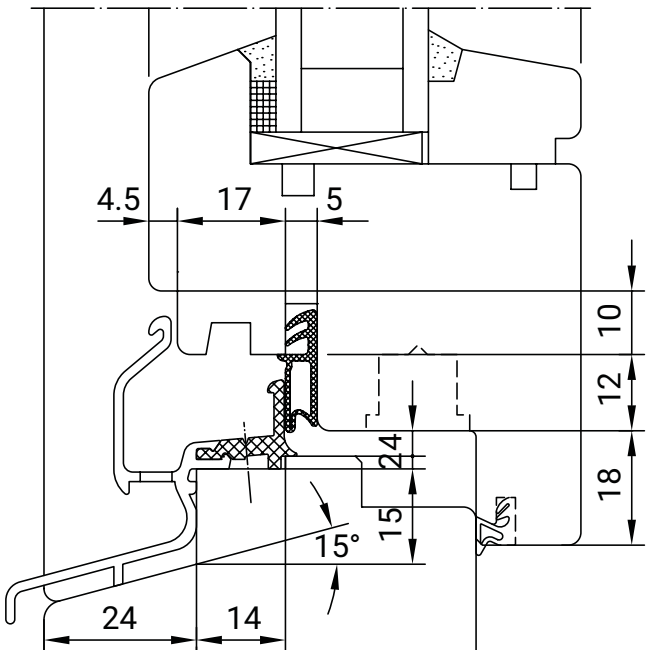
Einbaubeispiel GTR 22.44
